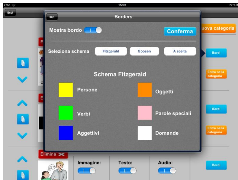
Figura 6. Finestra "Bordi"
